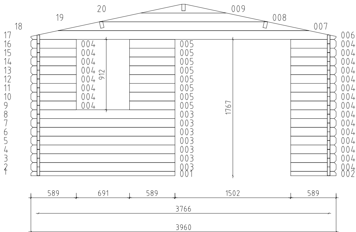
Façade avant
