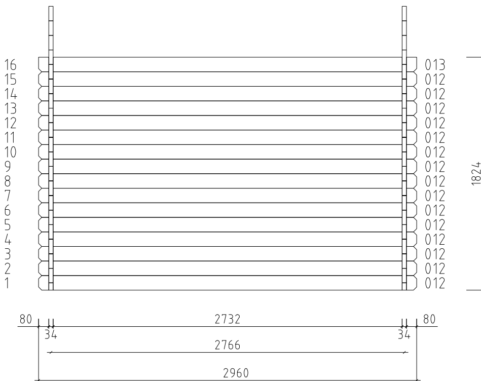
Façade latéral
