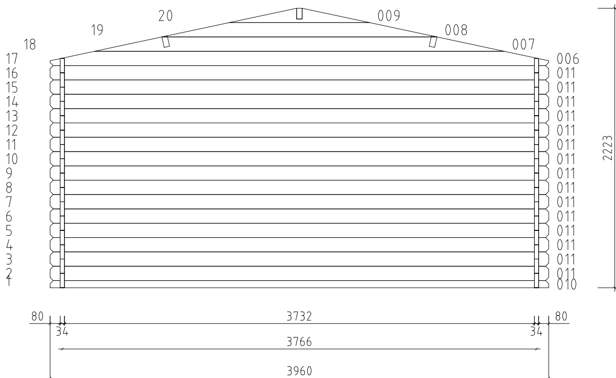
Façade arrière
