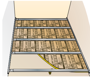
5 POSE DES FOURRURES VERTICALES
