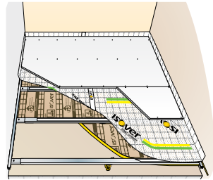
7 POSE DU PAREMENT
