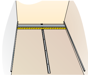
5 POSE DE LA LISSE ET FOURRURE MURALE
