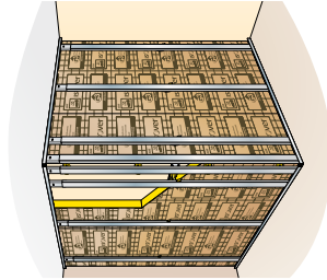
7 FOURRURES VERTICALES D'ANGLE AVEC CONNECTOR
