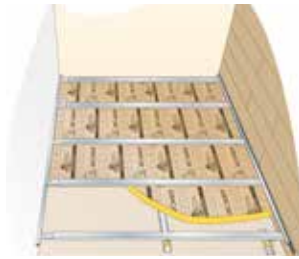
8 POSE DE L'ISOLANT ET FOURRURE
