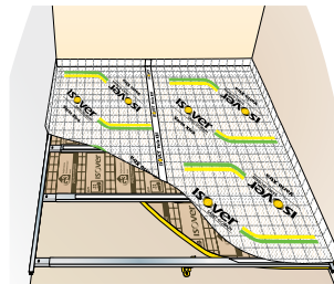
6 MEMBRANE VARIO X-TRA FIXÉE AU DOUBLE FACE
