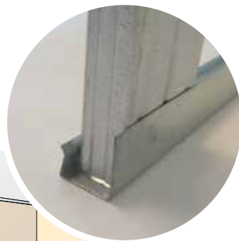
Lisses Clip'Optima basse et haute fixées au sol et au plafond.
