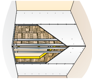
8 FINITION PLAQUE DE PLÂTRE
