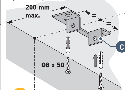
Chape fixée au plafond
