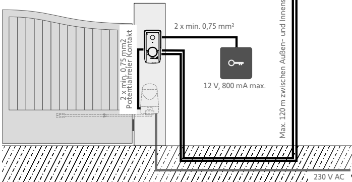
Kabel des Torantriebs
