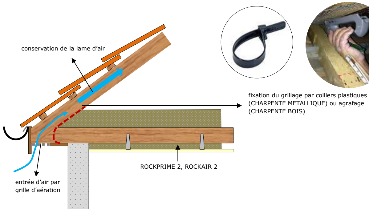
Figure 14 : Schéma de principe de la mise en œuvre du grillage de confinement sur une charpente industrielle en bois avec entrée d'air basse (type grille de ventilation en sous face du débord de toit)
