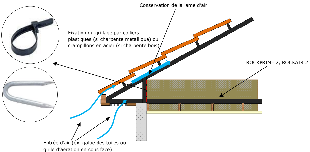
Figure 4 : Schéma de principe de la mise en œuvre du grillage de confinement sur une charpente industrielle métallique « petit entrain »
