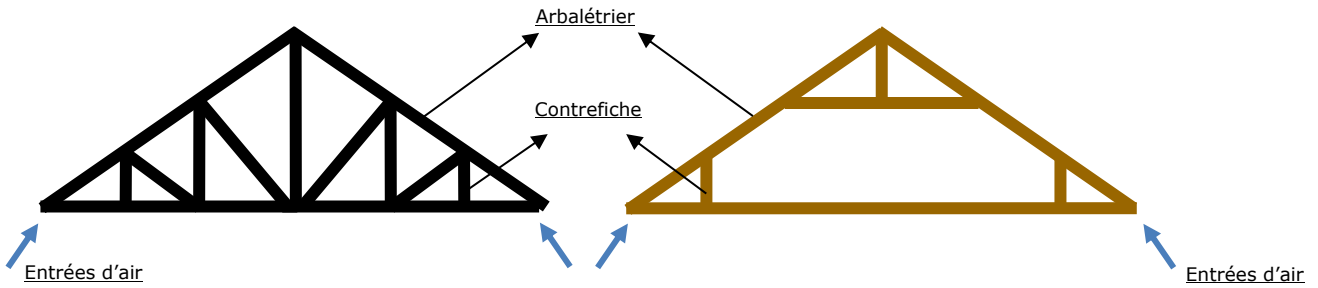
Figure 2 : Schéma de fermette de type « en N » en métal (gauche) et de type « à entrain retroussé » en bois (droite)
