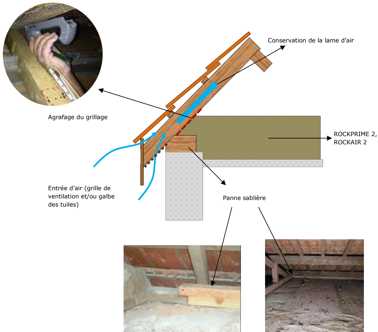
Figure 1 : Schéma de principe de la mise en œuvre du grillage de confinement sur une charpente traditionnelle
