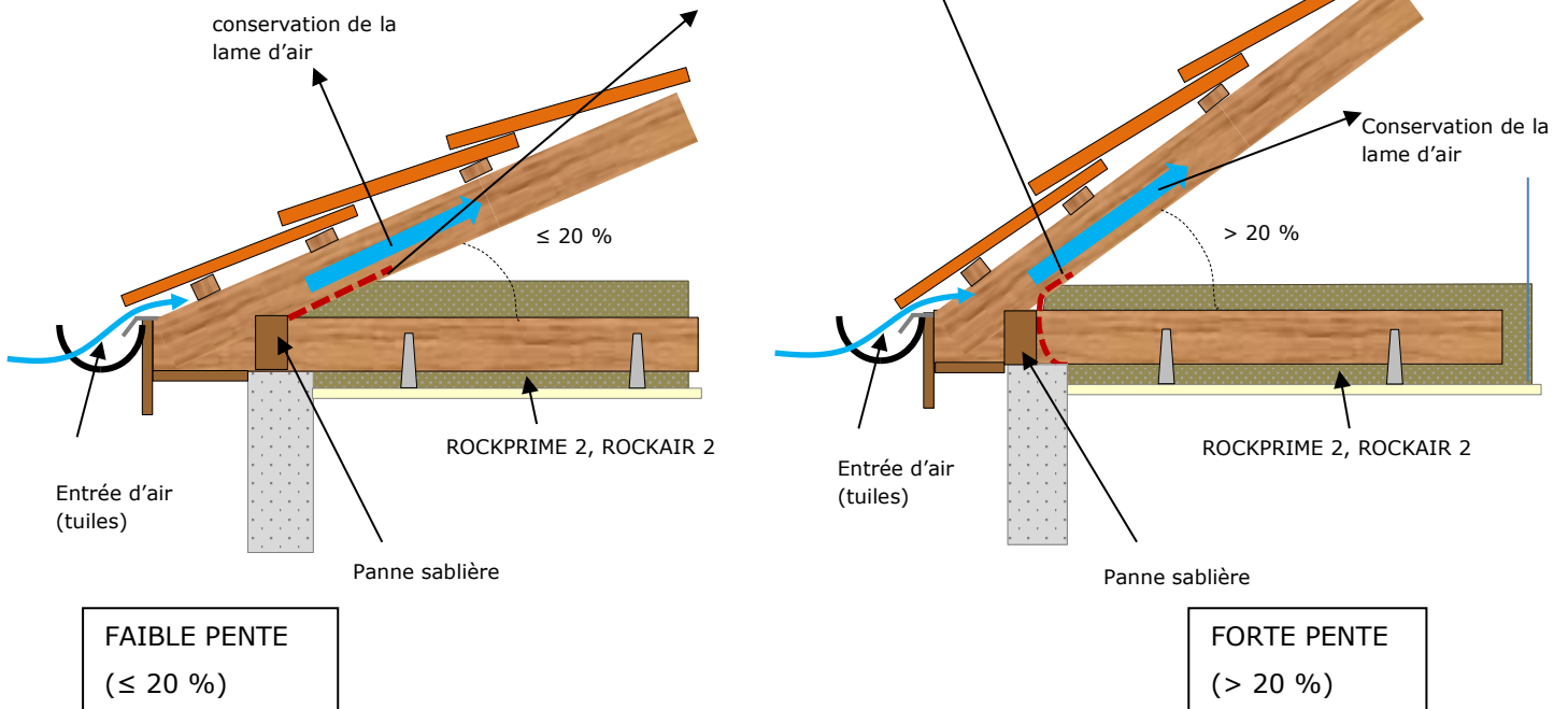
Figure 8 : Schéma de principe de la mise en œuvre du grillage de confinement sur une charpente industrielle en bois à faible pente (gauche) et à forte pente (droite) avec entrée d'air par le galbe des tuiles
