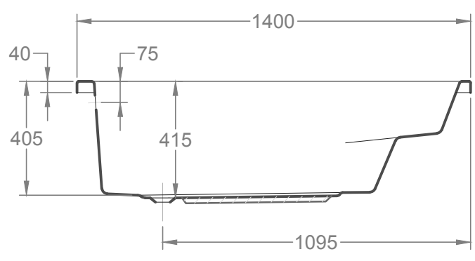
SEC: A-A
