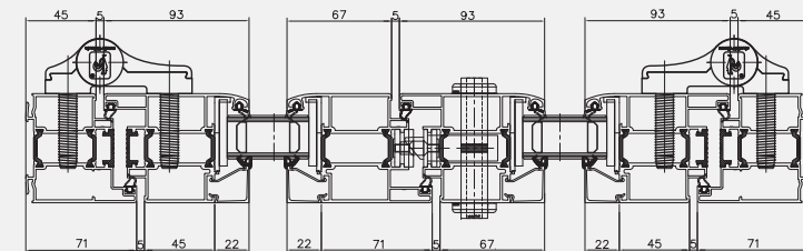
Coupe horizontale
