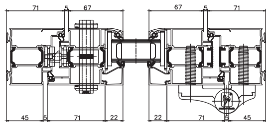
Coupe horizontale
